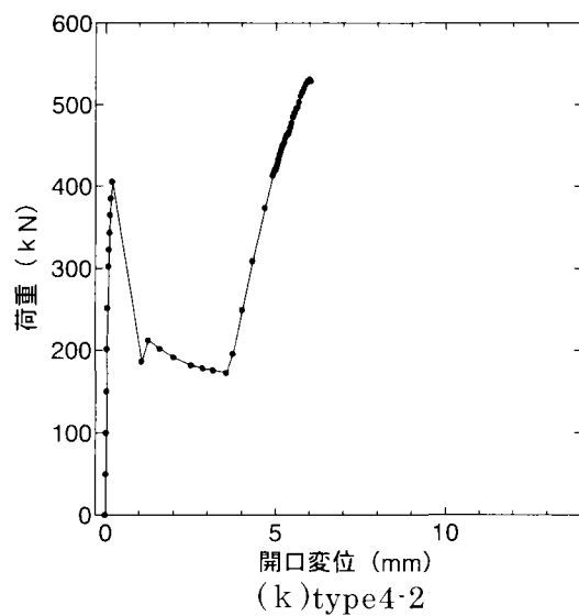
図 板厚 25mm(その 2)
