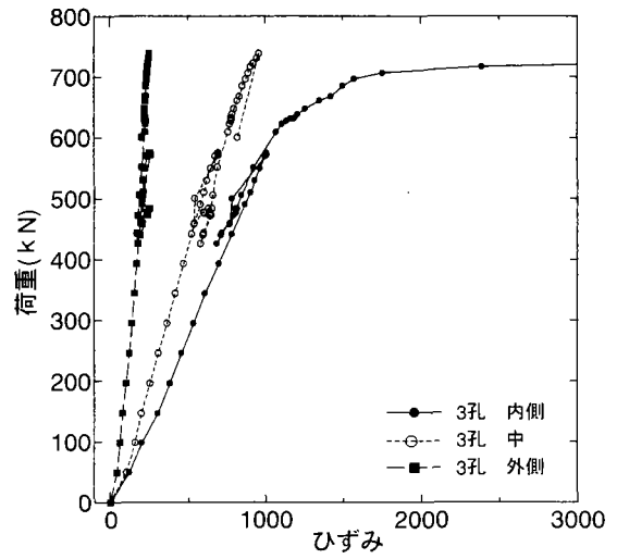
(b)板厚 25mm type1-3 ボルト頭側
