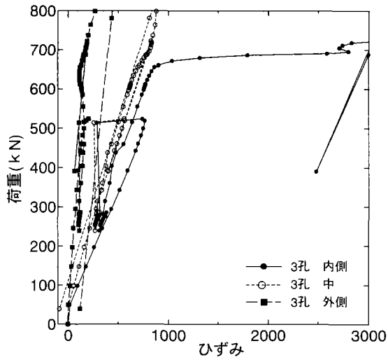
(g)板厚 25mm type4-3 ナット側
