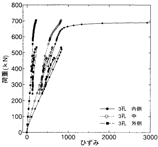
(i)板厚 25mm type5-3 ナット側
