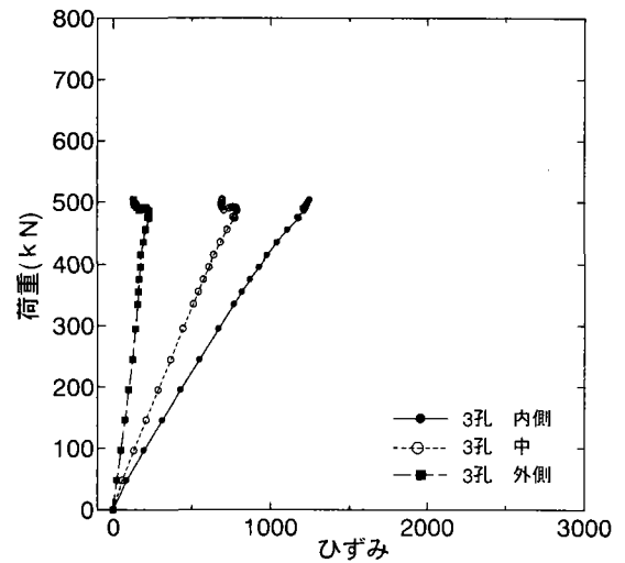
(b)板厚 16mm type1-3 ボルト頭側
