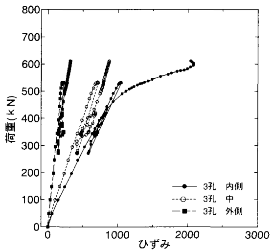
(f)板厚 22mm type3-3 ボルト頭側
