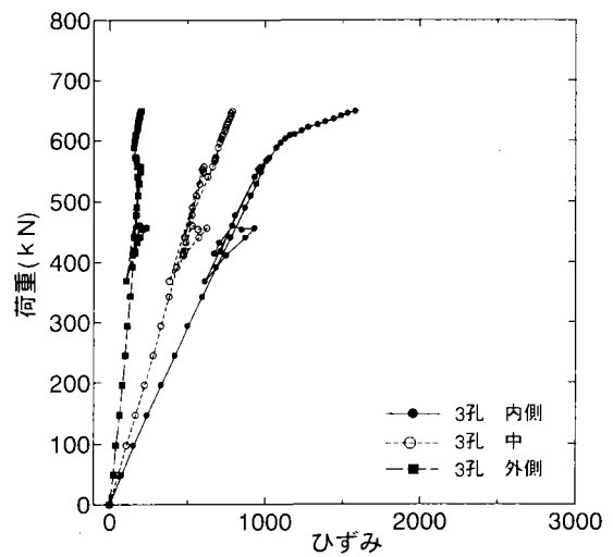
(b)板厚 22mm type1-3 ボルト頭側
