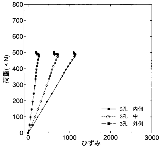
(a)板厚 16mm type1-3 ナット側
