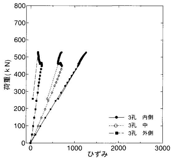
(e)板厚 16mm type3-3 ナット側
