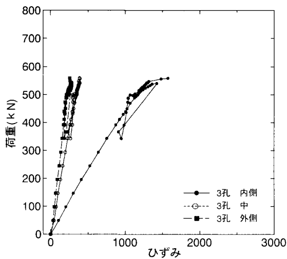
(a)板厚 19mm type1-3 ナット側
