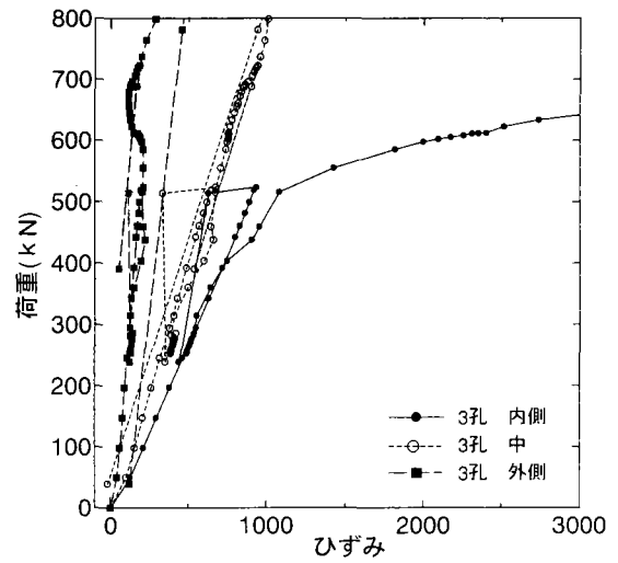
(h)板厚 25mm type4-3 ボルト頭側
