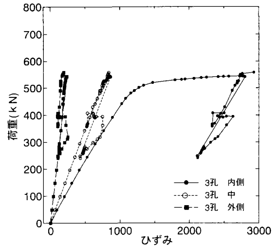
(h)板厚 19mm type5-3 ボルト頭側
