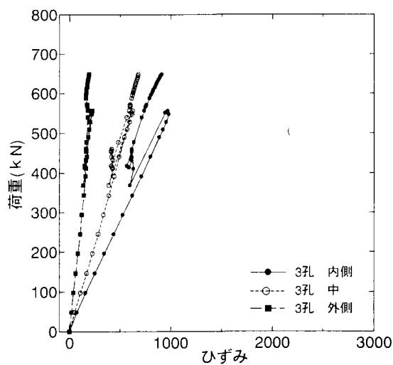
(a)板厚 22mm type1-3 ナット側
