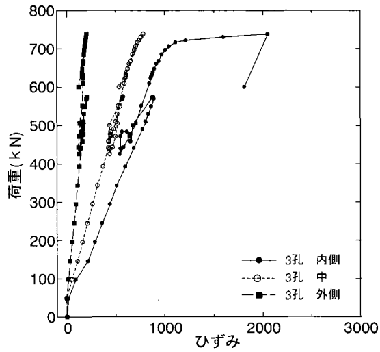
(a)板厚 25mm type1-3 ナット側
