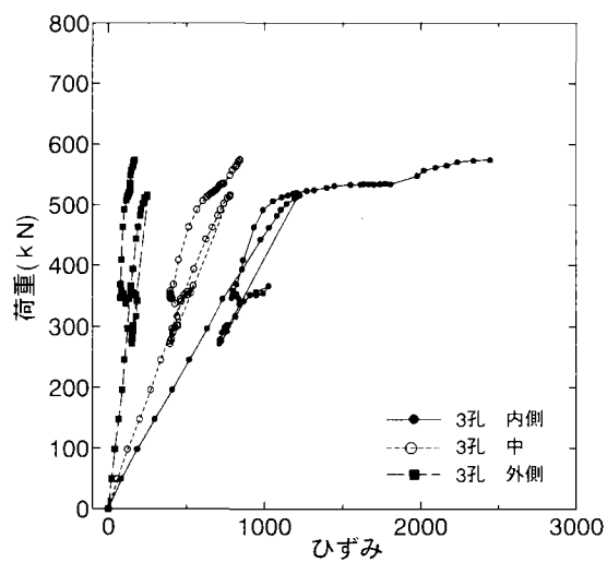
(c)板厚 19mm type2-3 ナット側
