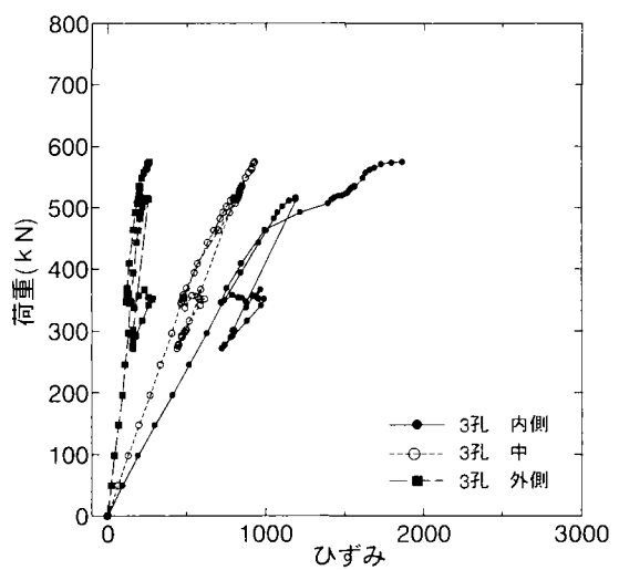
(d)板厚 19mm type2-3 ボルト頭側
