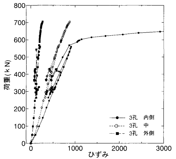
(f)板厚 25mm type3-3 ボルト頭側
