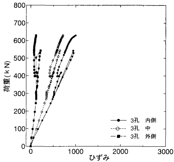
(c)板厚 22mm type2-3 ナット側
