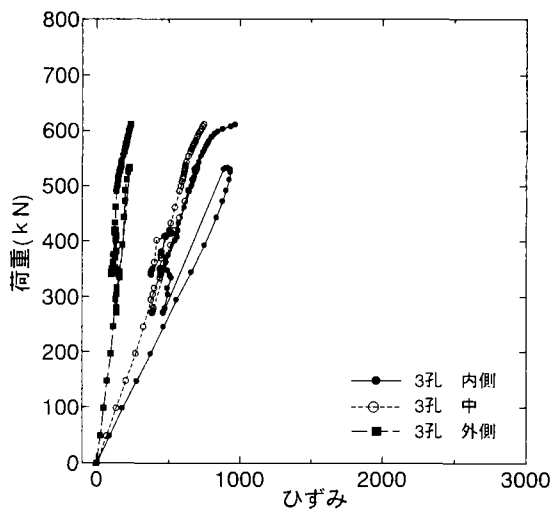
(e)板厚 22mm type3-3 ナット側
