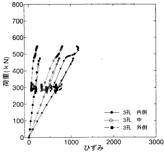
(e)板厚 19mm type3-3 ナット側
