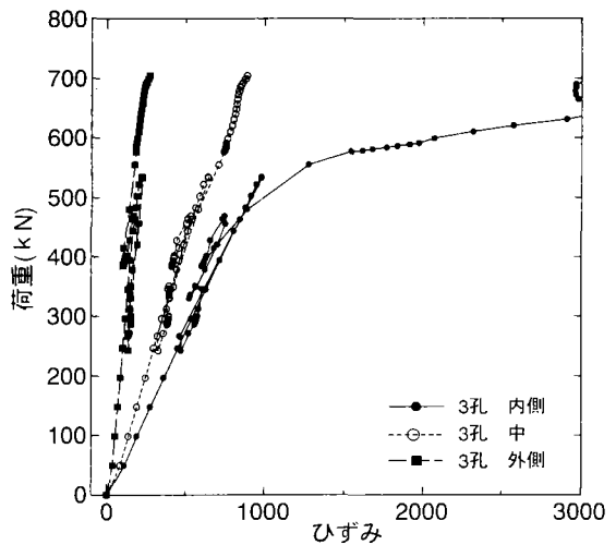
(j)板厚 25mm type5-3 ボルト頭側
