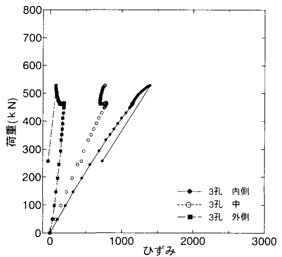
(f)板厚 16mm type3-3 ボルト頭側
