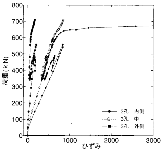
(k)板厚 25mm type6-3 ナット側
