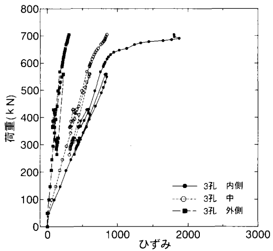
(e)板厚 25mm type3-3 ナット側
