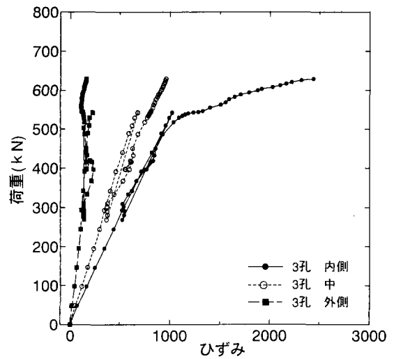
(d)板厚 22mm type2-3 ボルト頭側
