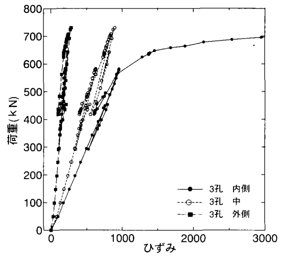
(d)板厚 25mm type2-3 ボルト頭側
