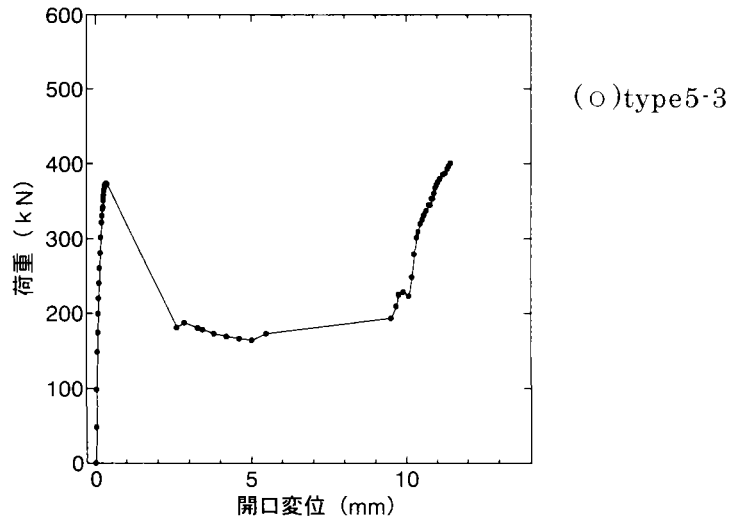
板厚 16mm(その4)
