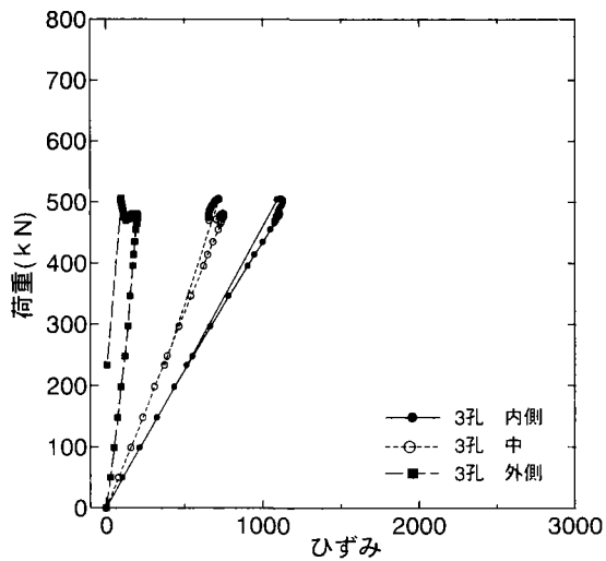
(g)板厚 16mm type5-3 ナット側
