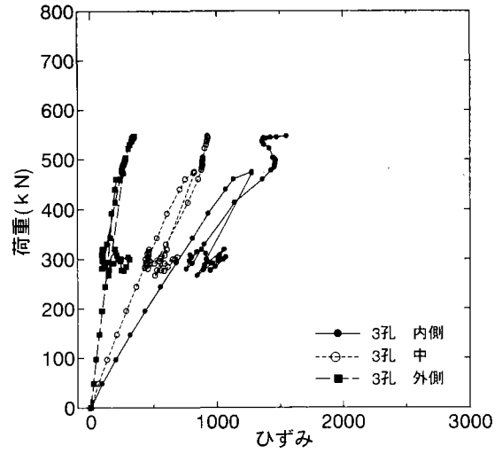
(f)板厚 19mm type3-3 ボルト頭側
