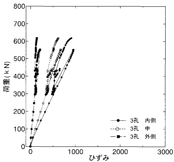
(g)板厚 22mm type5-3 ナット側
