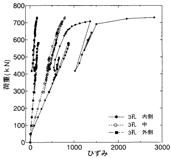
(c)板厚 25mm type2-3 ナット側
