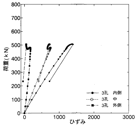
(h)板厚 16mm type5-3 ボルト頭側
