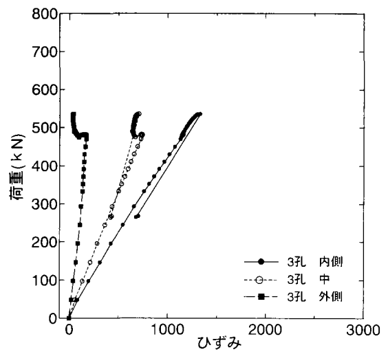
(d)板厚 16mm type2-3 ボルト頭側
