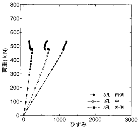
(c)板厚 16mm type2-3 ナット側
