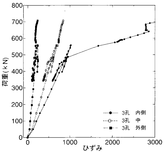
(l)板厚 25mm type6-3 ボルト頭側
