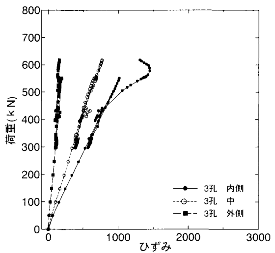
(h)板厚 22mm type5-3 ボルト頭側
