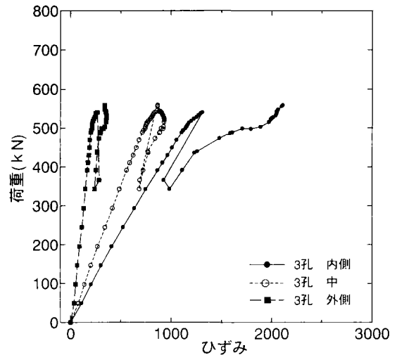
(b)板厚 19mm type1-3 ボルト頭側
