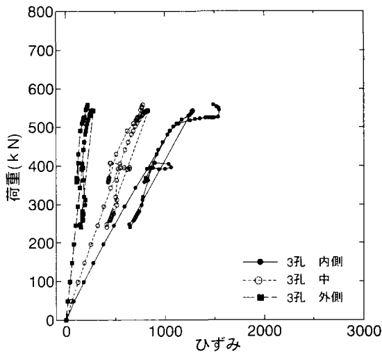
(g)板厚 19mm type5-3 ナット側
